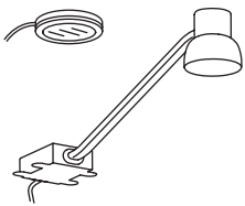
OMLOPP faretto a LED o illuminazione a LED per mobile* Diametro del faretto rotondo: cm 6,8. Colore: bianco, alluminio e nero.
