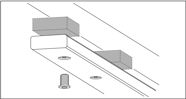
Illustration détaillée montrant comment compenser la hauteur sous plafond avec des pièces intermédiaires.
