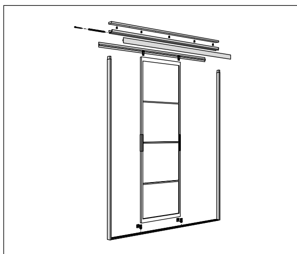
Illustration détaillée des éléments du système SKYTТА lorsque les portes sont parfaitement adaptées.
