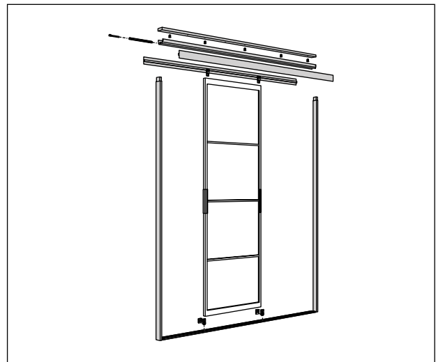
Detaillierte Darstellung der SKYTТА Systemteile, wenn die Türen perfekt passen.
